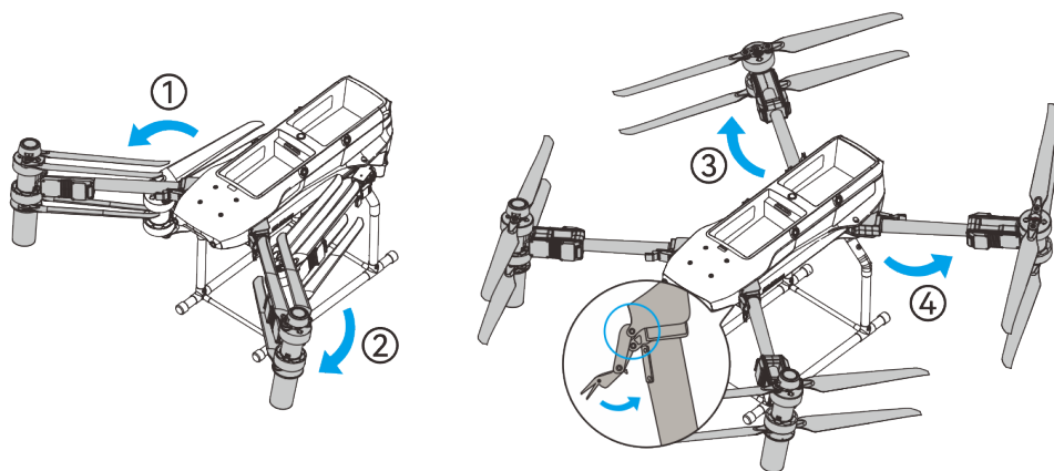
图 3-7 展开并固定机臂
