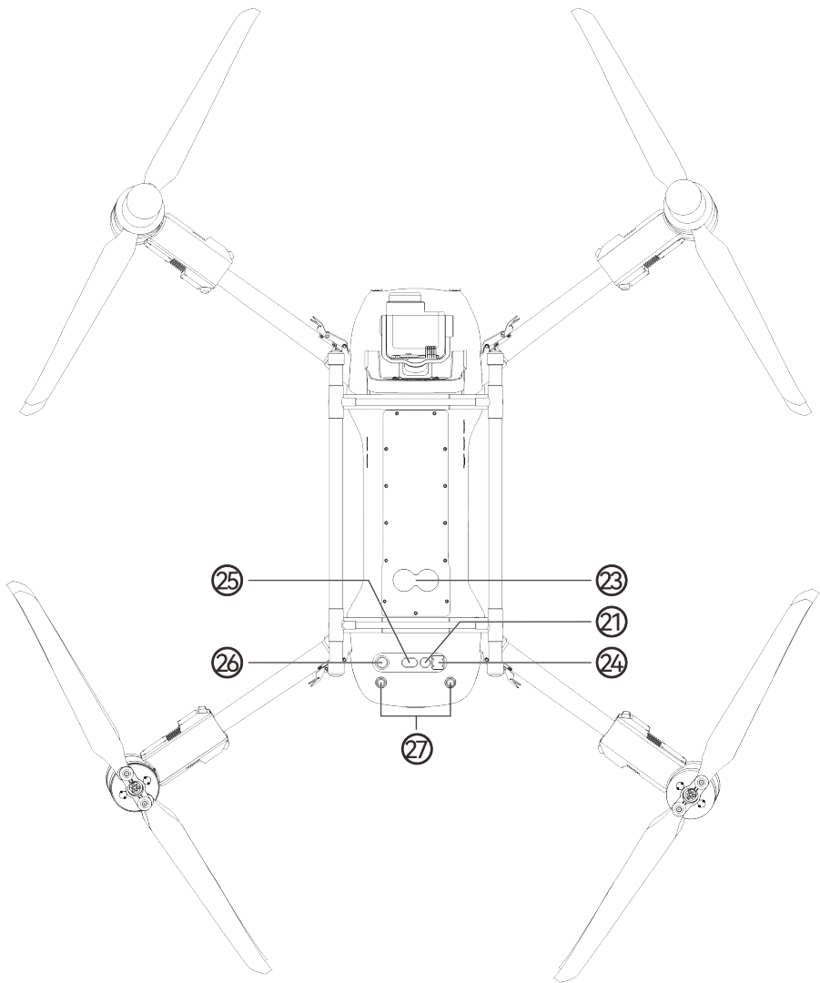
图 3-5 飞行器底视图
