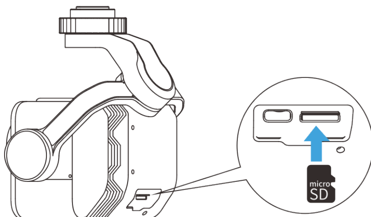
图 3-18 安装 microSD 卡
