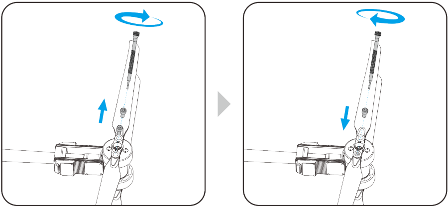
图 3-9 螺旋桨安装示意图
