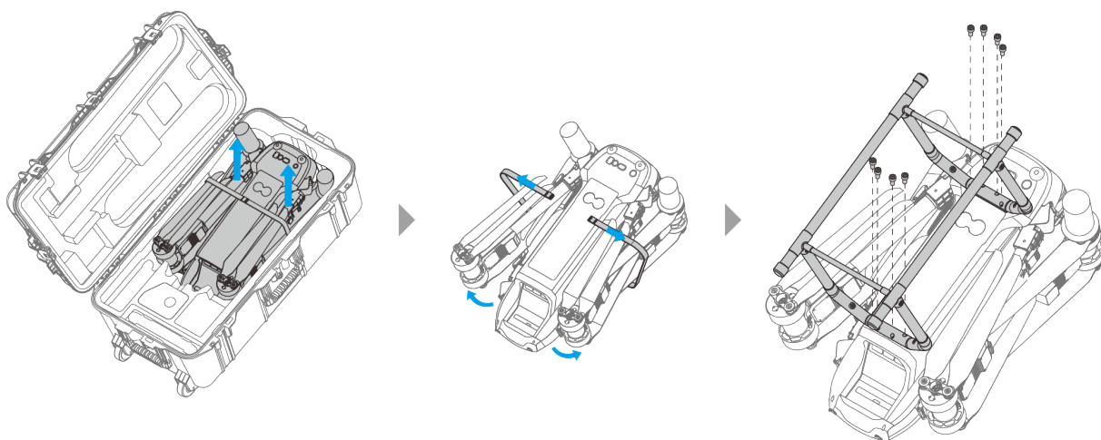
图 3-6 安装飞行器脚架
