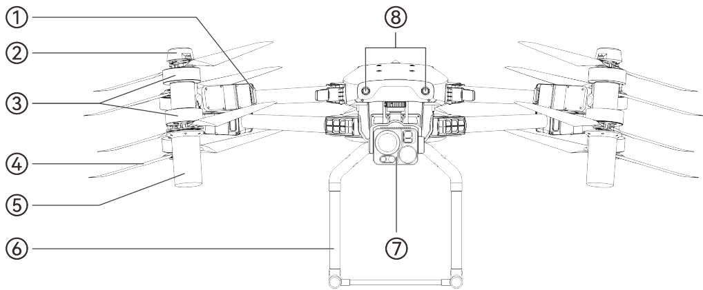
图 3-1 飞行器正视图
