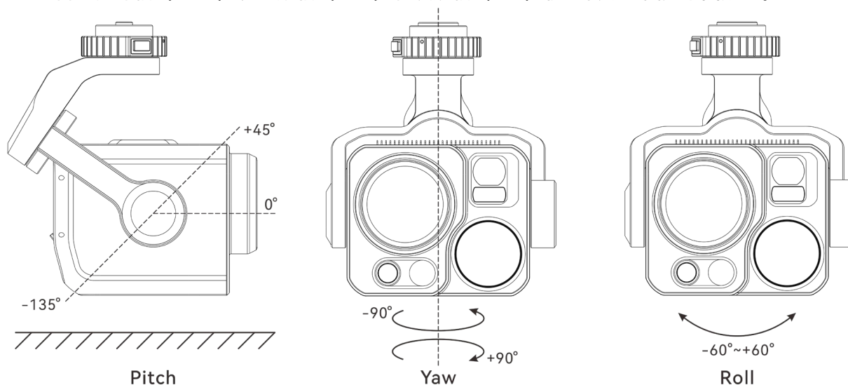
图 3-15 DG-L35T 云台相机机械转动范围
