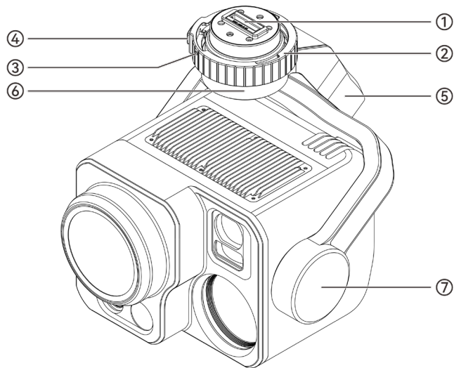
图 3-14 云台结构
