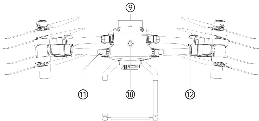
图 3-2 飞行器后视图
