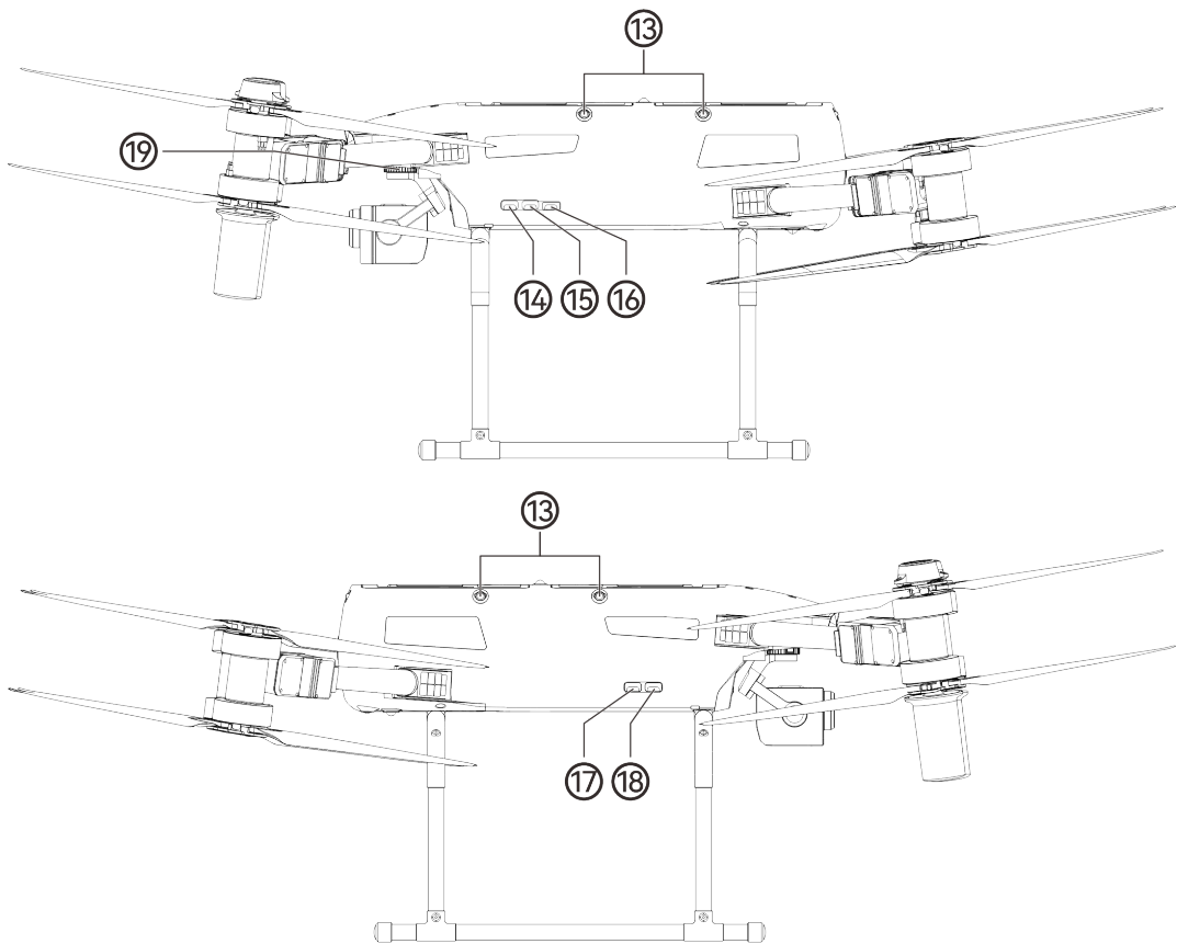
图 3-3 飞行器侧视图
