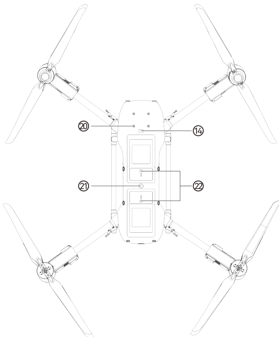
图 3-4 飞行器顶视图
