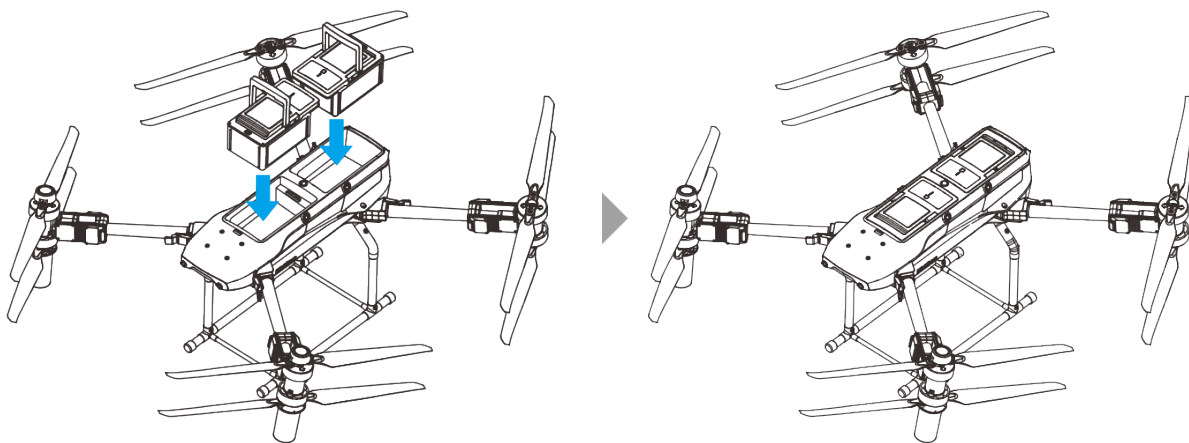
图 5-2 安装智能电池
