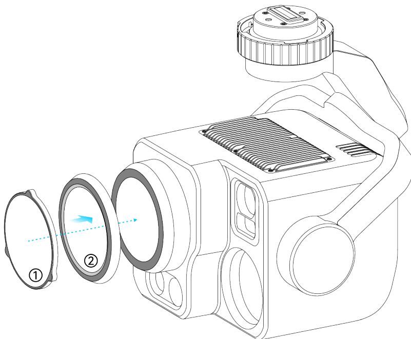
图 3-17 安装 ND 镜
