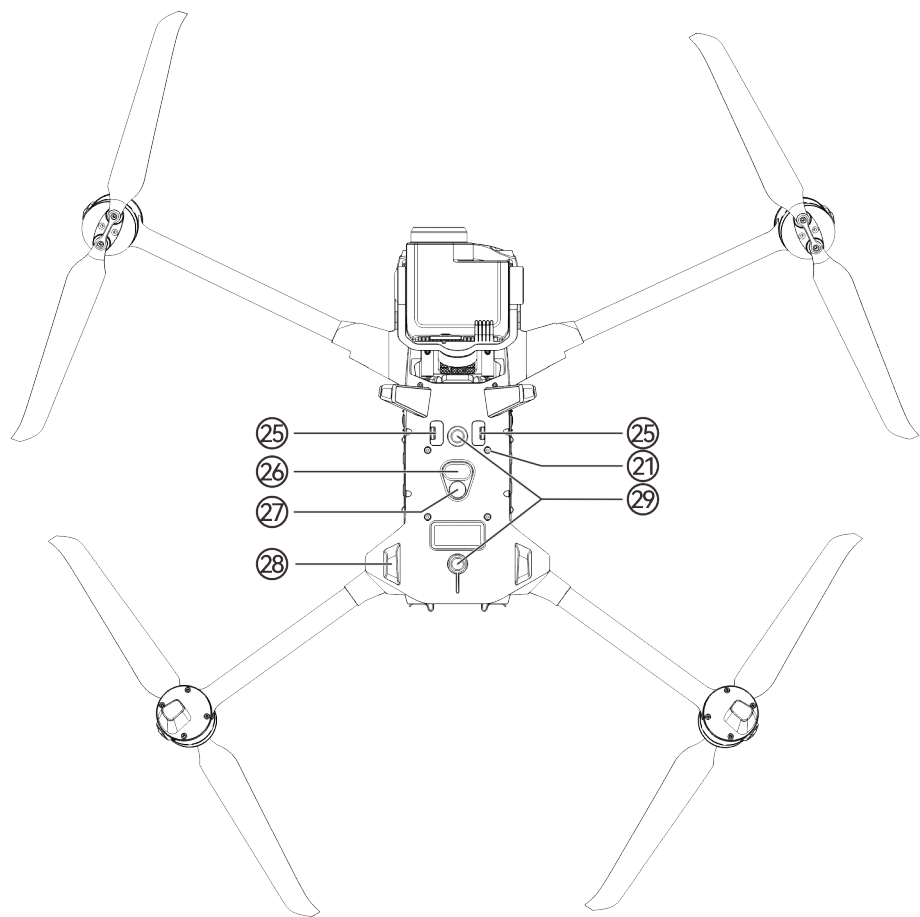
图 3-5 无人机底视图
