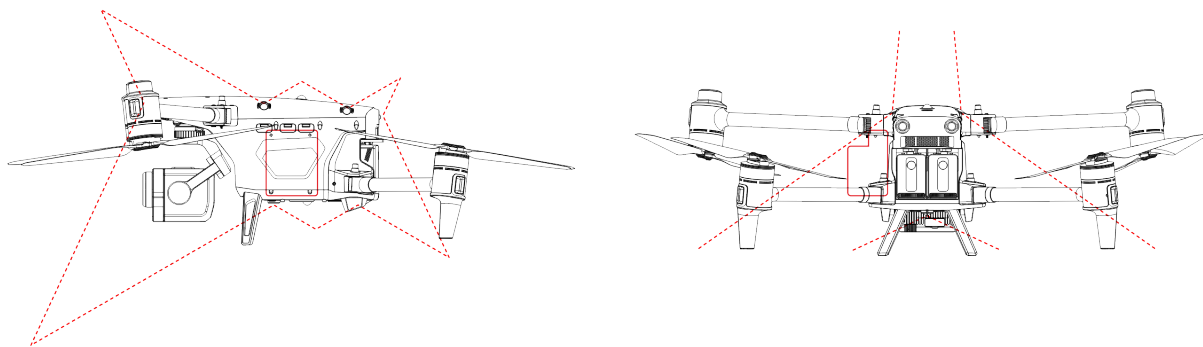
图 2-1 安全区域（虚线内为非干涉区域）
