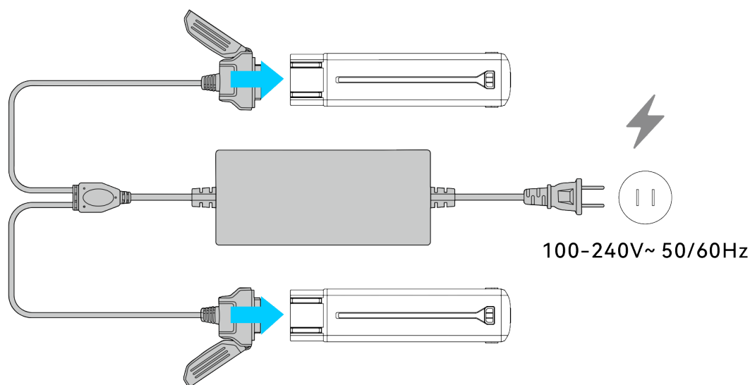
图 5-7 通过电池充电器给智能电池充电
