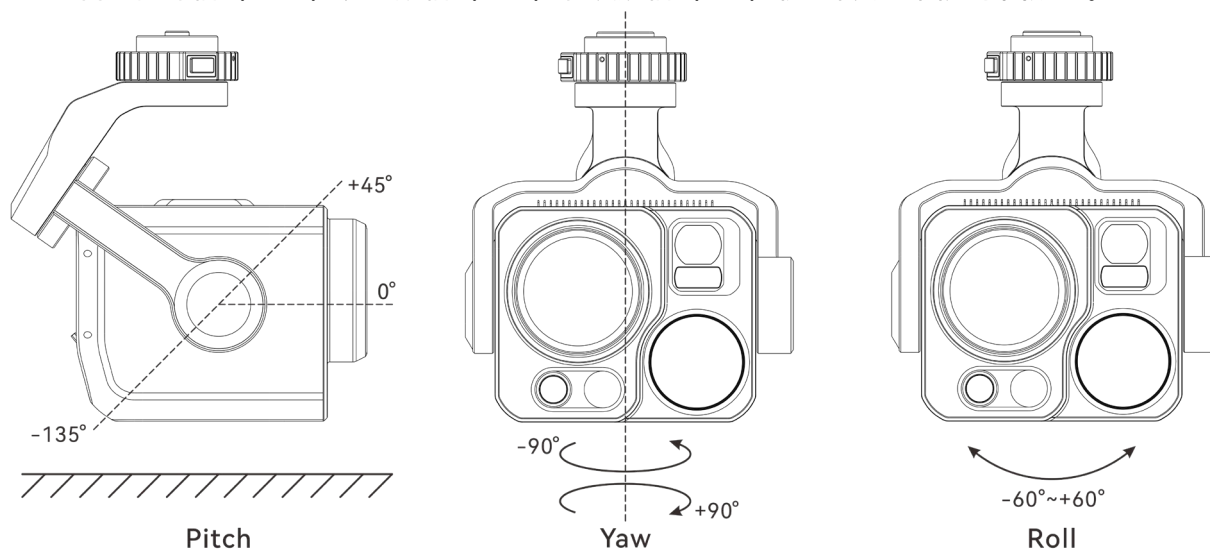
图 3-14 L35T 云台机械转动范围
