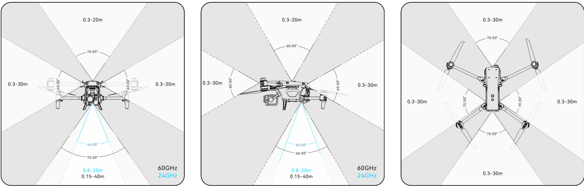
图 2-4 毫米波观测范围
