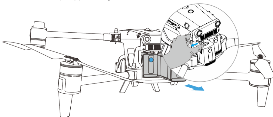
图 5-3 取出智能电池
