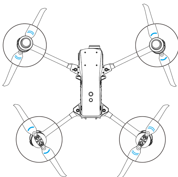
图 3-6 无人机螺旋桨安装布局（丝印标识均朝向机身顶部）
