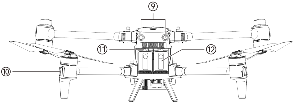
图 3-2 无人机后视图
