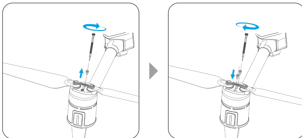
图 3-7 螺旋桨安装示意图
