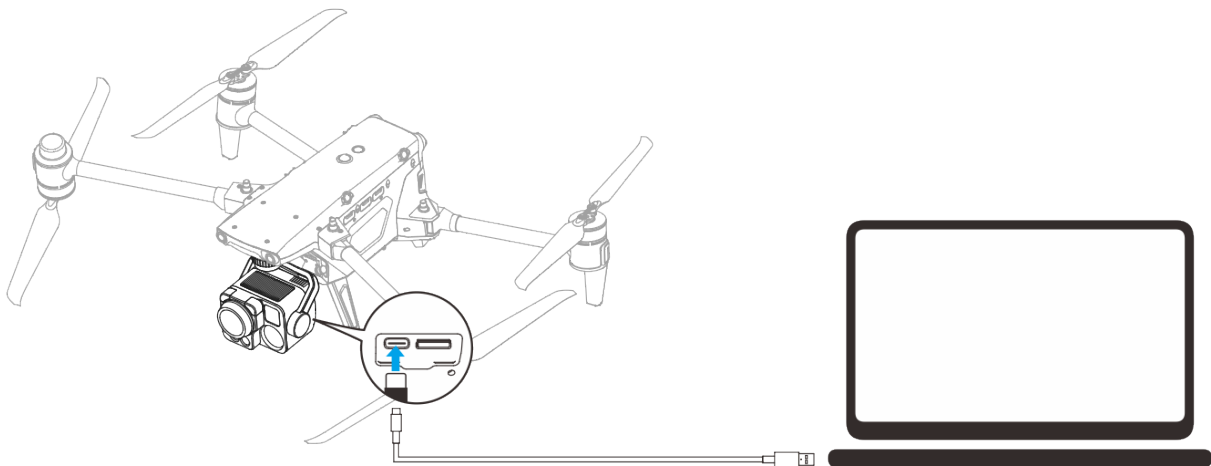
图 3-18 通过云台 USB-C 接口连接至计算机
