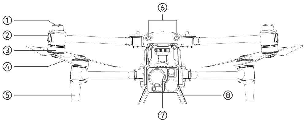
图 3-1 无人机正视图
