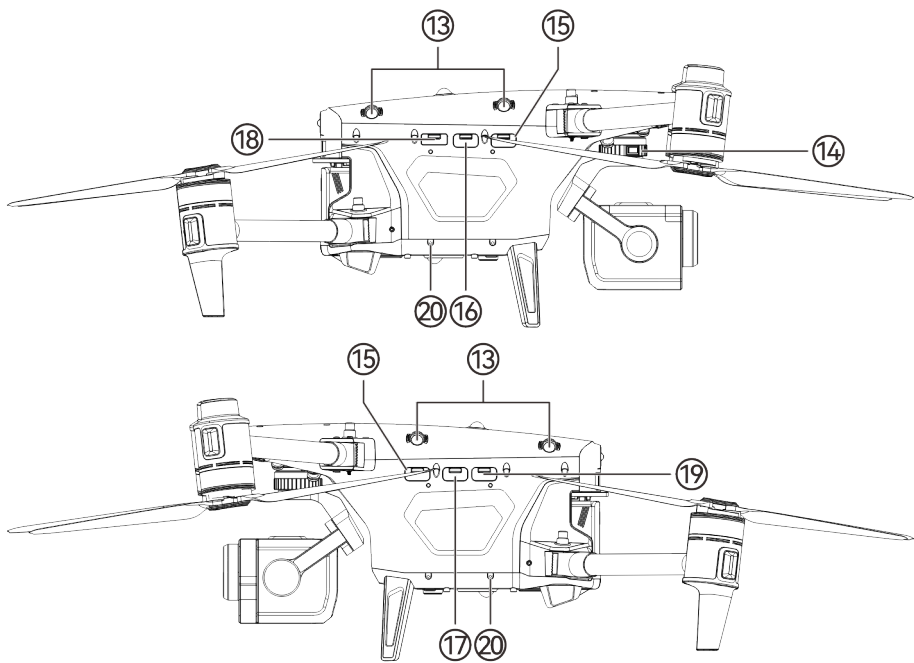
图 3-3 无人机侧视图
