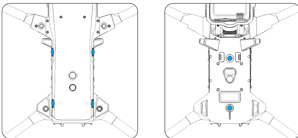
图 2-3 无人机左上侧、右上侧和底部视觉避障镜头组
