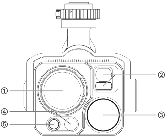
图 3-12 L35T 云台相机布局
