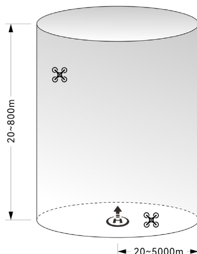
圖 2-5 限高限遠示意圖
