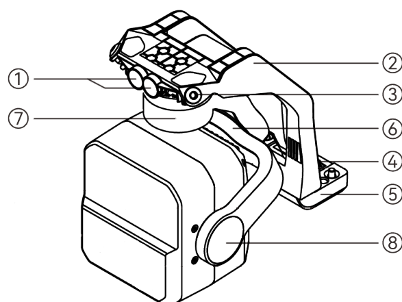
圖 3-11 雲臺結構
