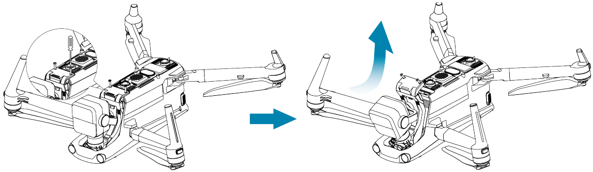
圖 3-13 拆卸雲臺
