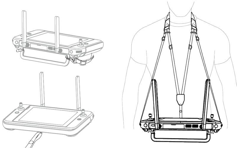
圖 4-4 安裝遙控器掛帶（按需）
