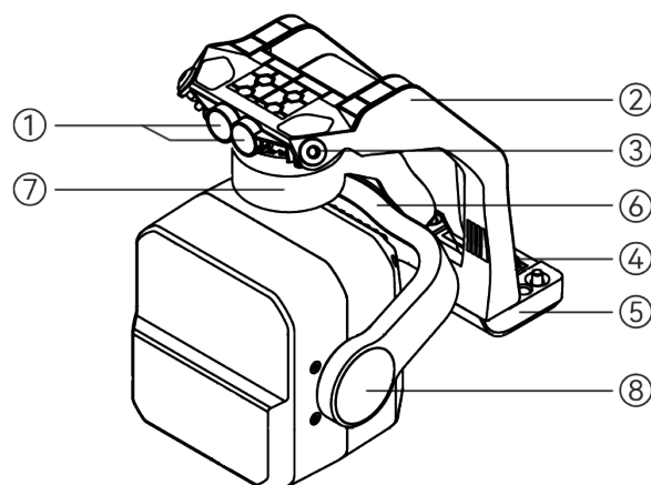
圖 3-11 雲臺結構
