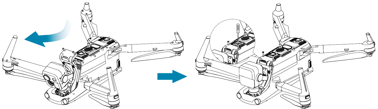
圖 3-14 安裝云台
